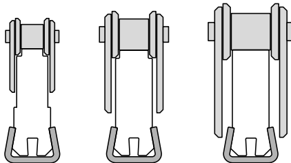
#40 ANSI
