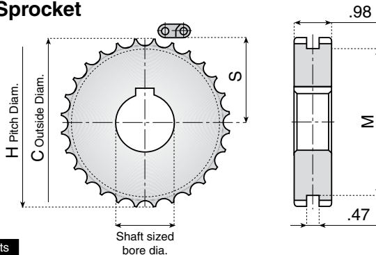
Drive Sprocket
